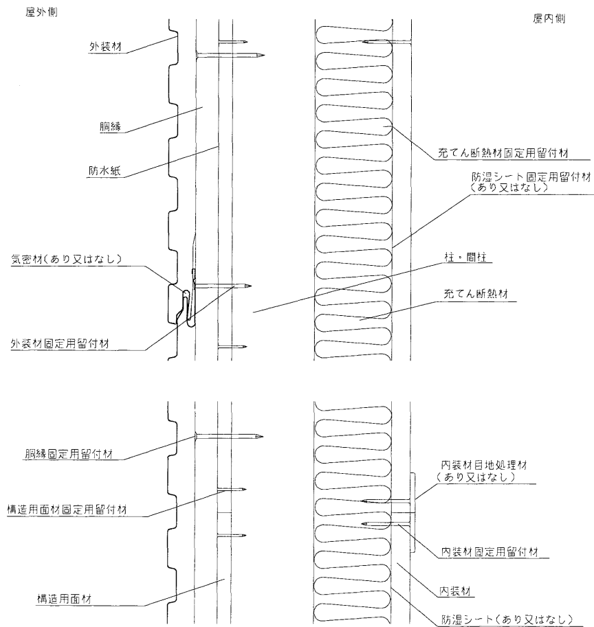
鉛直断面図
