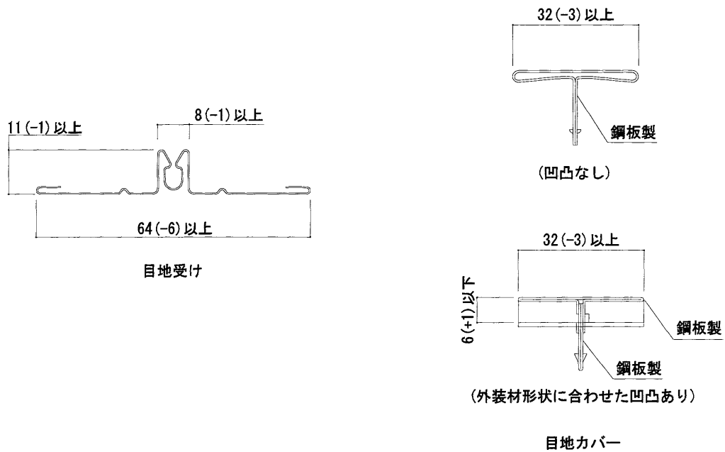
役物断面形状図
