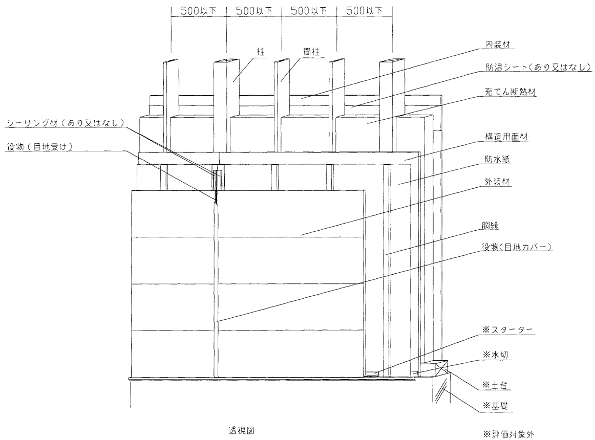
透視図
