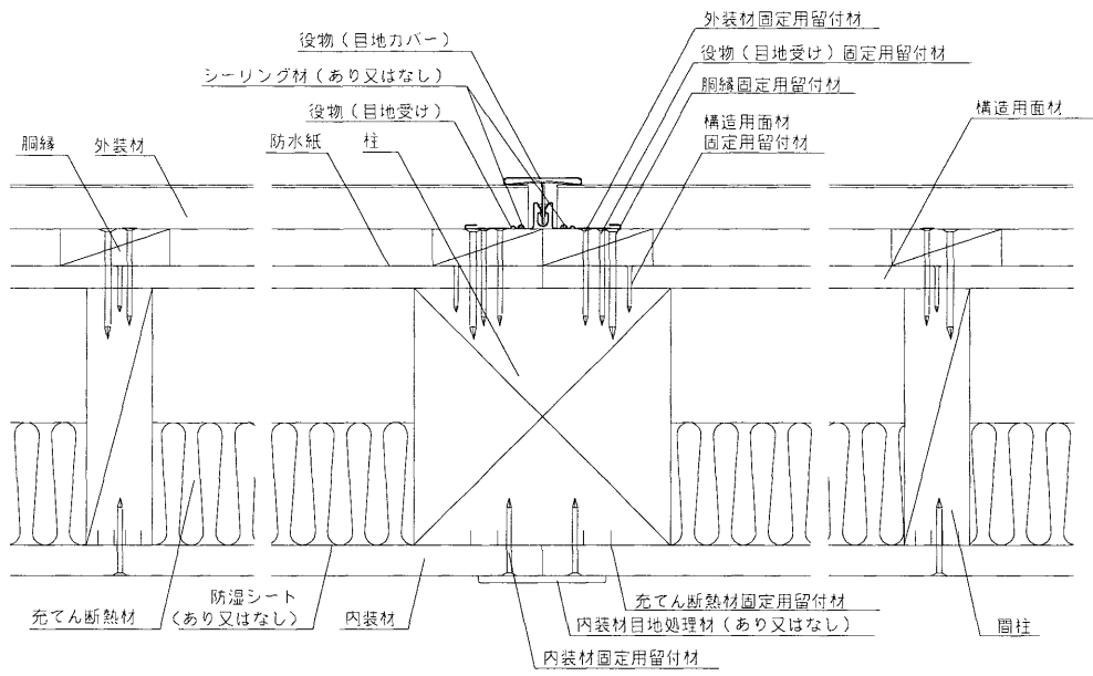
水平断面図
