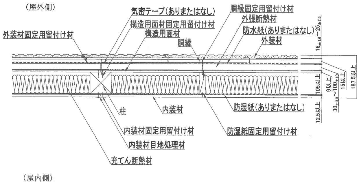
水平断面図(縦張の場合)
