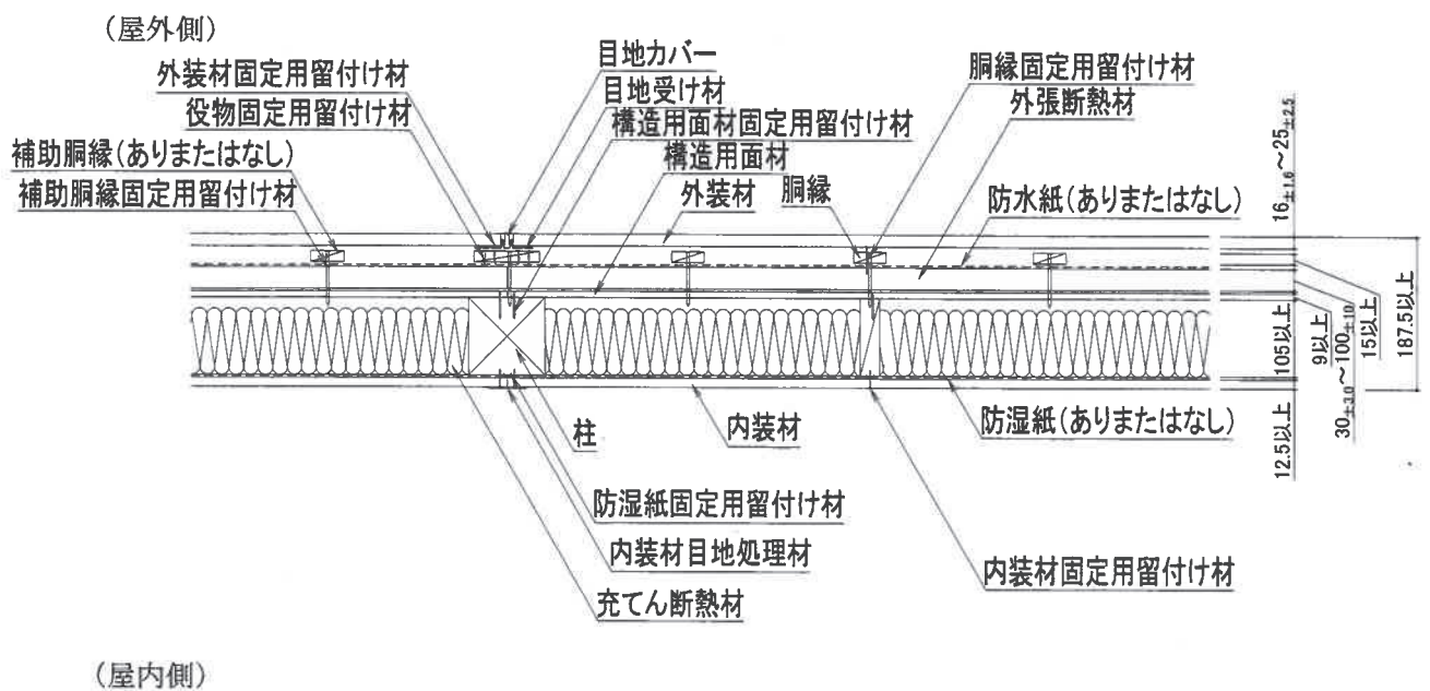
水平断面図 (横張の場合)
