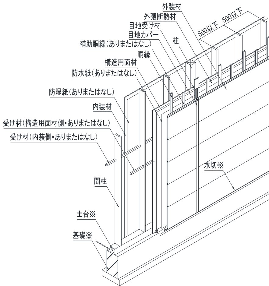
斜視図(外装材：横張の場合)
