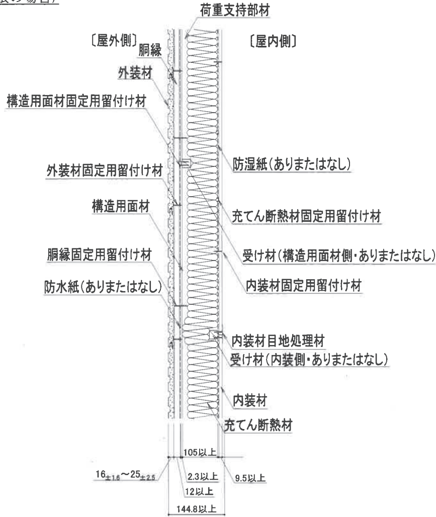
目地部詳細図 (横張の場合の場合・役物：水密材 B あり仕様)
