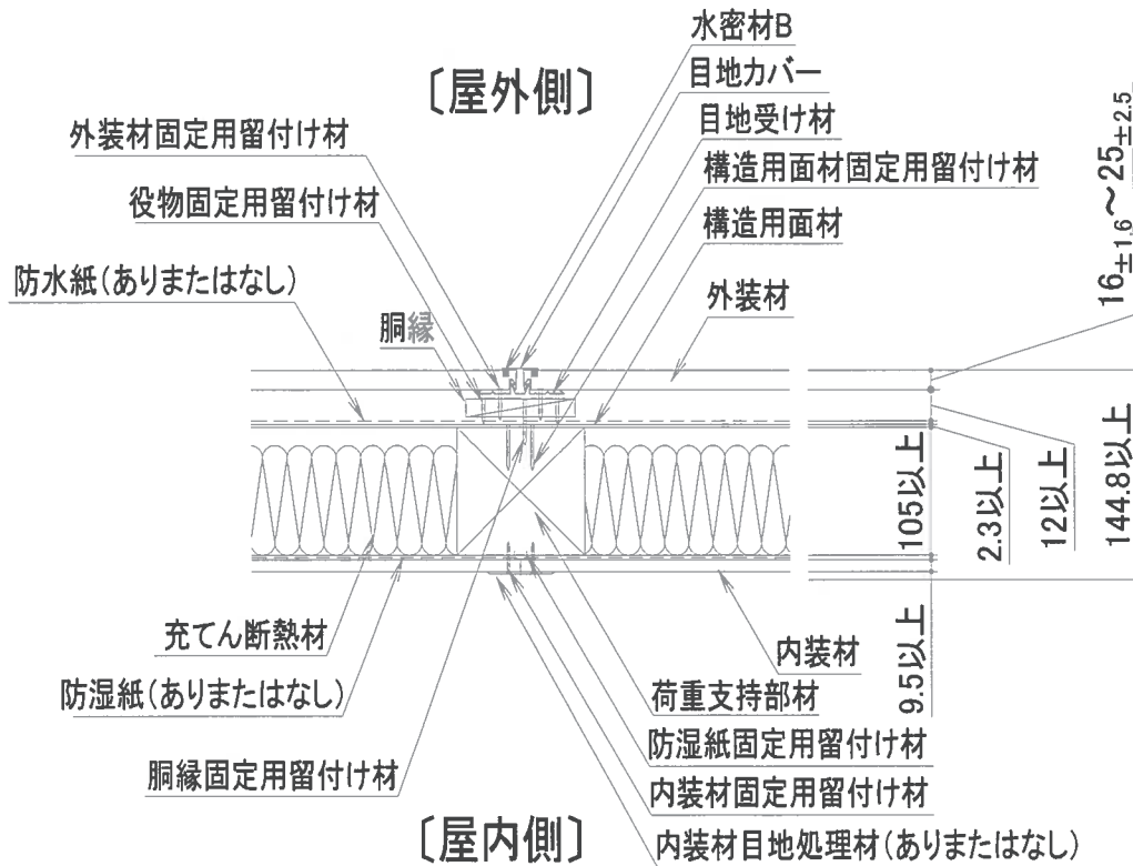
目地部詳細図 (横張の場合の場合・役物：水密材 B あり仕様)
