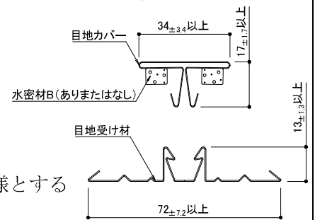
目地カバーと目地受け材の代表例
