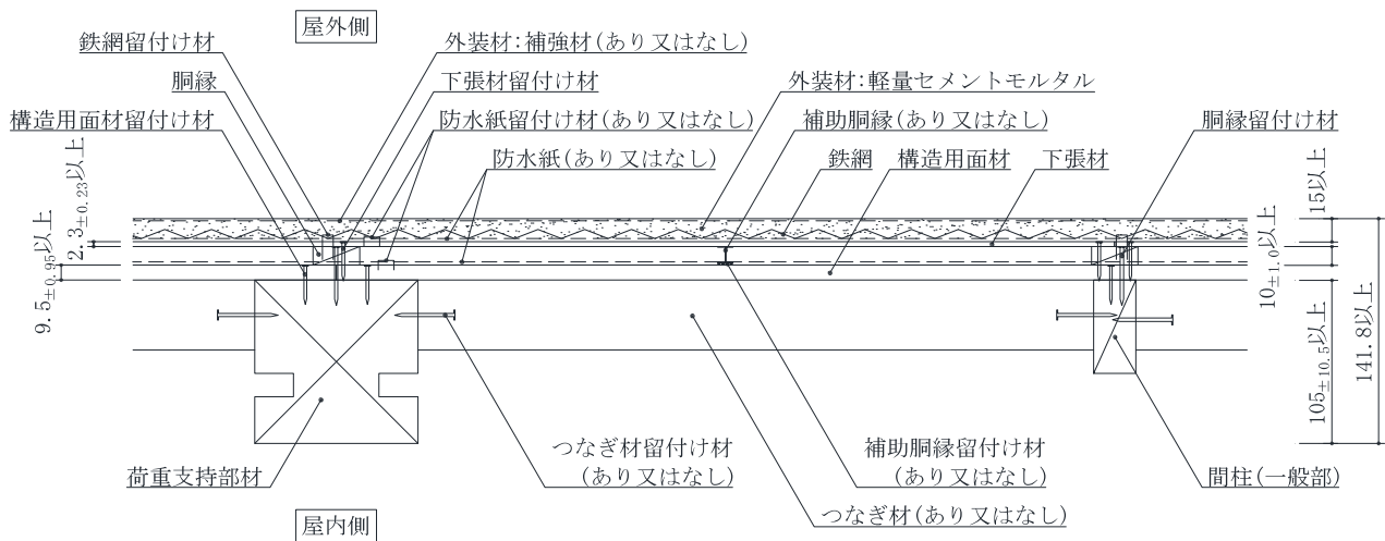
水平断面詳細図
