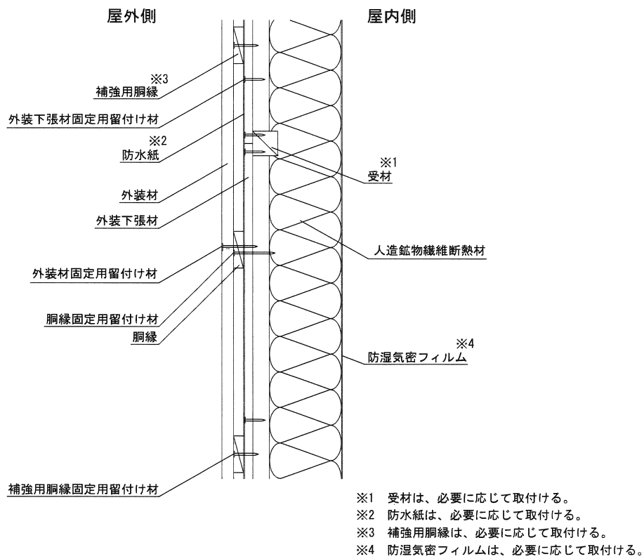
図-6 断面図 (外装材横張仕様 (胴縁 横張))
